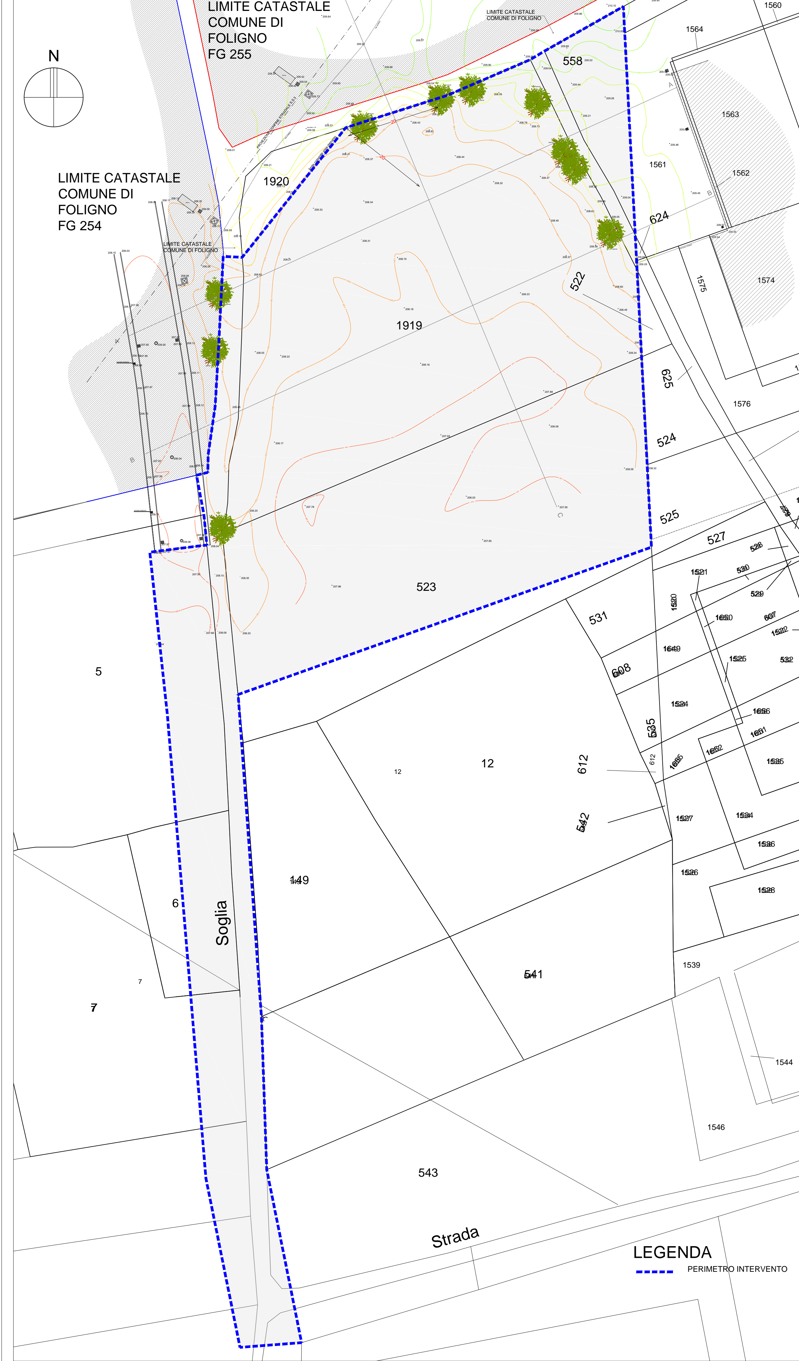
PLANIMETRIA GENERALE - PIANO QUOTATO
